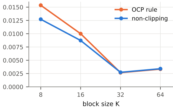
RepVGG-A0, e4m3
