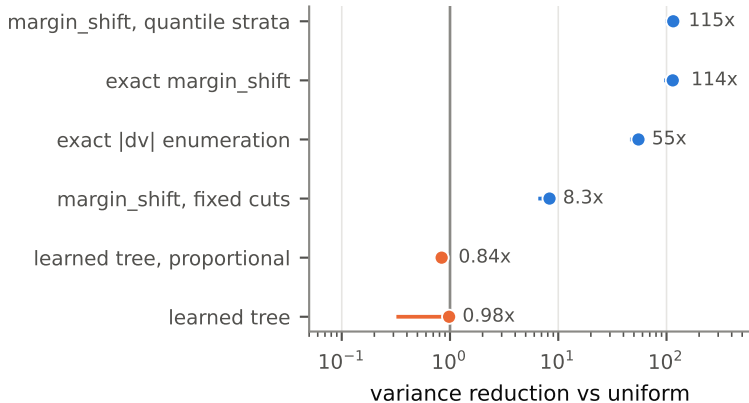
ResNet8, e3m2
