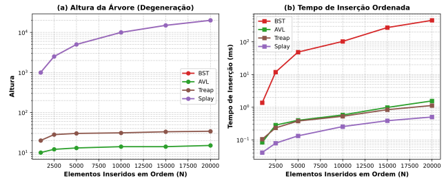
Figura 7: Cenário 2: Degeneração da BST vs estabilidade AVL/Treap.
