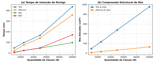
Figura 6: Cenário 1: Desempenho e compressão na Trie vs Patricia.
