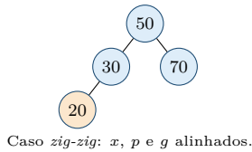
Figura 3: Rastreamento do passo autoajustável homogêneo ( zig-zig ) na Árvore Splay: (1) acesso à chave profunda 20 com nós alinhados à esquerda ( x = 20, p = 30, g = 50 ); (2) primeira rotação à direita aplicada sobre o avô g ; e (3) segunda rotação à direita sobre o pai p , promovendo a chave consultada à raiz e reduzindo pela metade a profundidade de todos os nós do caminho de busca.
