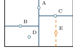
Figura 5: Rastreamento de particionamento e hierarquia espacial bidimensional ( k = 2 ) na KD-Tree: (1) hierarquia da árvore com alternância cíclica de eixos de corte ( x na profundidade par, y na ímpar); (2) subdivisão do plano euclidiano antes de E ; e (3) inserção do ponto E(7.5, 2.0) delimitando um novo hiperplano ortogonal restrito à sub-região de seus ancestrais.
