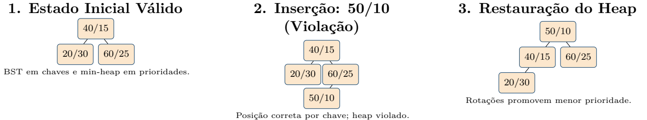
Figura 4: Rastreamento de inserção e rebalanceamento via min-heap na Árvore Treap: (1) estado inicial perfeitamente balanceado obedecendo à ordem simétrica e ao min-heap; (2) inserção em folha da chave 50 com prioridade estocástica de alta precedência ( p = 10 ), violando o min-heap frente ao pai ( p = 25 ); e (3) rotações ascendentes à esquerda que promovem 50/10 à raiz, restaurando simultaneamente ambas as invariantes.
