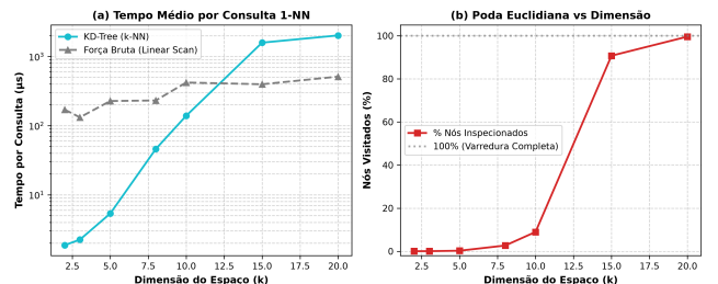
Figura 9: Cenário 4: Tempo de consulta k -NN e nós visitados vs dimensão ( k \in [2, 20] ). A KD-Tree é 91,1 \times superior em 2D, mas a perda de poda em altas dimensões ( k \geq 15 ) torna a busca linear 4,0 \times mais rápida.
