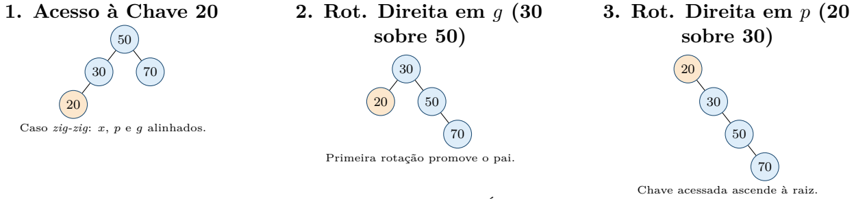
Figura 3: Rastreamento do passo autoajustável homogêneo ( zig-zig ) na Árvore Splay: (1) acesso à chave profunda 20 com nós alinhados à esquerda ( x = 20, p = 30, g = 50 ); (2) primeira rotação à direita aplicada sobre o avô g ; e (3) segunda rotação à direita sobre o pai p , promovendo a chave consultada à raiz e reduzindo pela metade a profundidade de todos os nós do caminho de busca.
