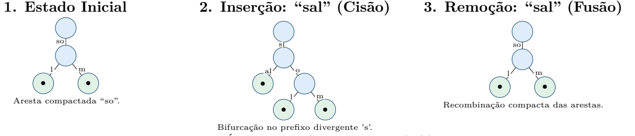
Figura 2: Rastreamento de mutação estrutural na Árvore Patricia (Radix compactada): (1) estado inicial com aresta compactada "so" e folhas terminais; (2) inserção de "sal" provocando a cisão atômica da aresta no maior prefixo comum (LCP = "s") com novo nó bifurcador; e (3) remoção de "sal" com fusão reversa de arestas, restabelecendo o rótulo consolidado original.
