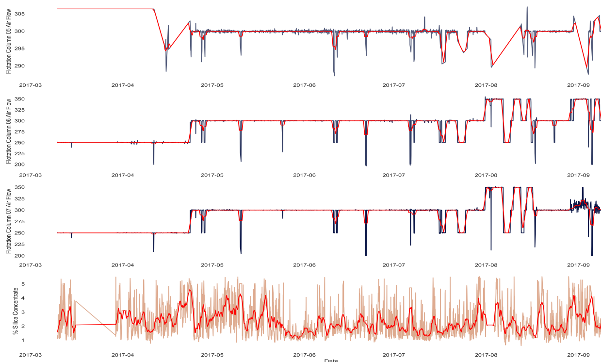
Figura 12: Em ordem crescente (cima para baixo) as séries temporais do fluxo de ar das colunas 5, 6 e 7 de flotação. Por último a série temporal para a concentração de sílica final.
