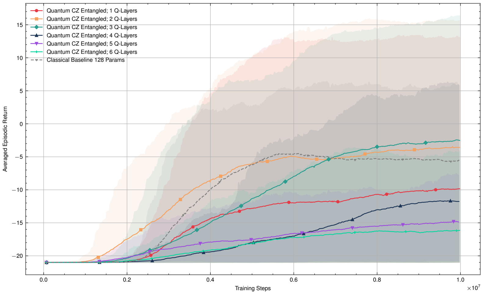
Episodic Return: Quantum CZ Entangled vs Classical Baseline 128 Params
