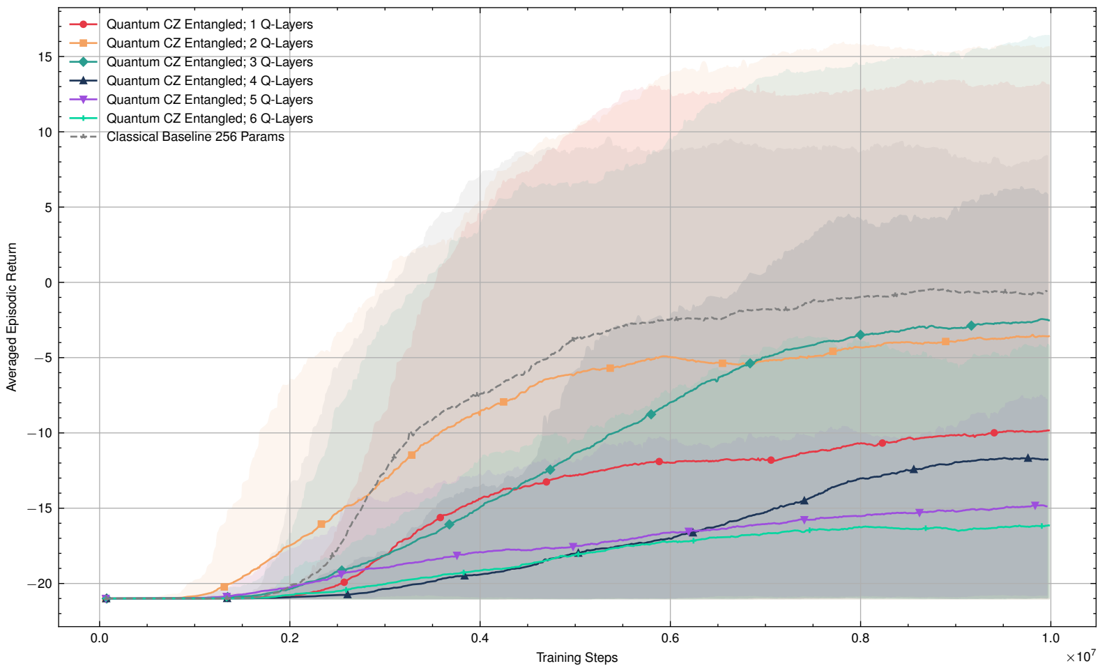
Episodic Return: Quantum CZ Entangled vs Classical Baseline 256 Params
