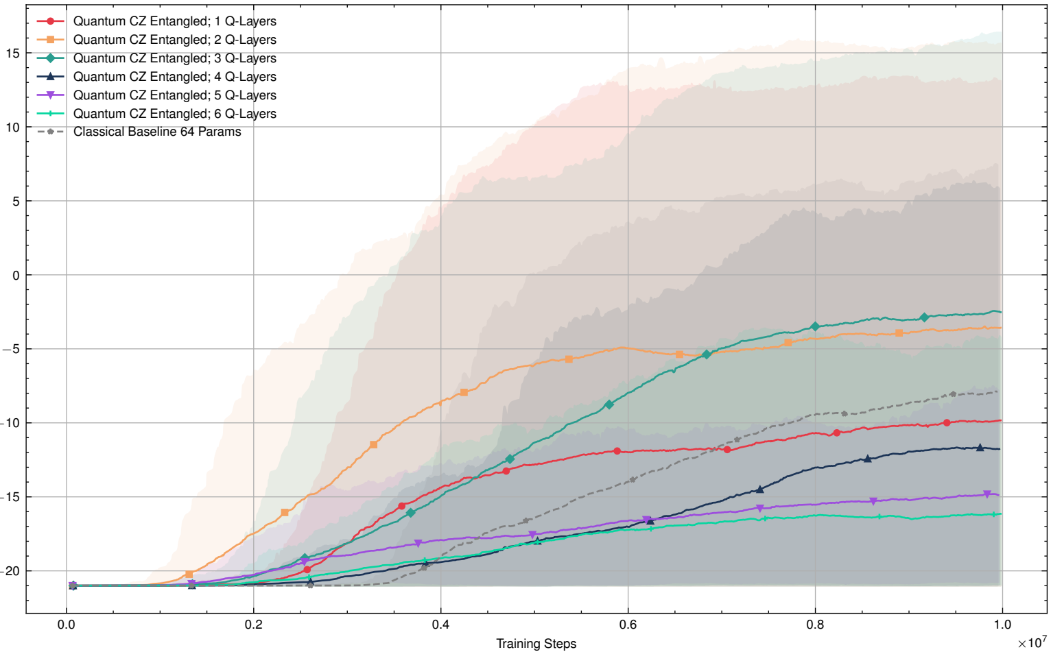
Episodic Return: Quantum CZ Entangled vs Classical Baseline 64 Params
