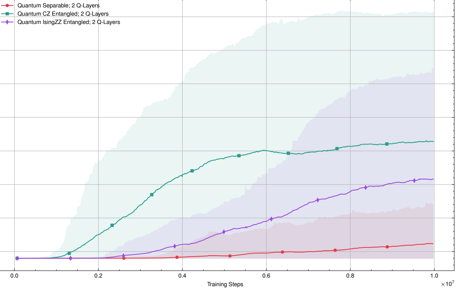
Episodic Return Comparison for 2 Q-Layers
