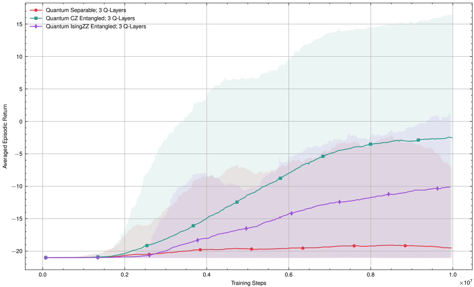
Episodic Return Comparison for 3 Q-Layers
