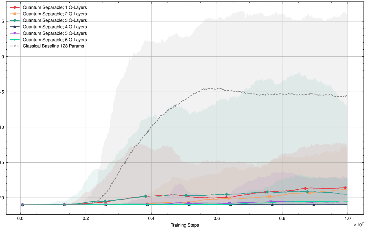
Episodic Return: Quantum Separable vs Classical Baseline 128 Params
