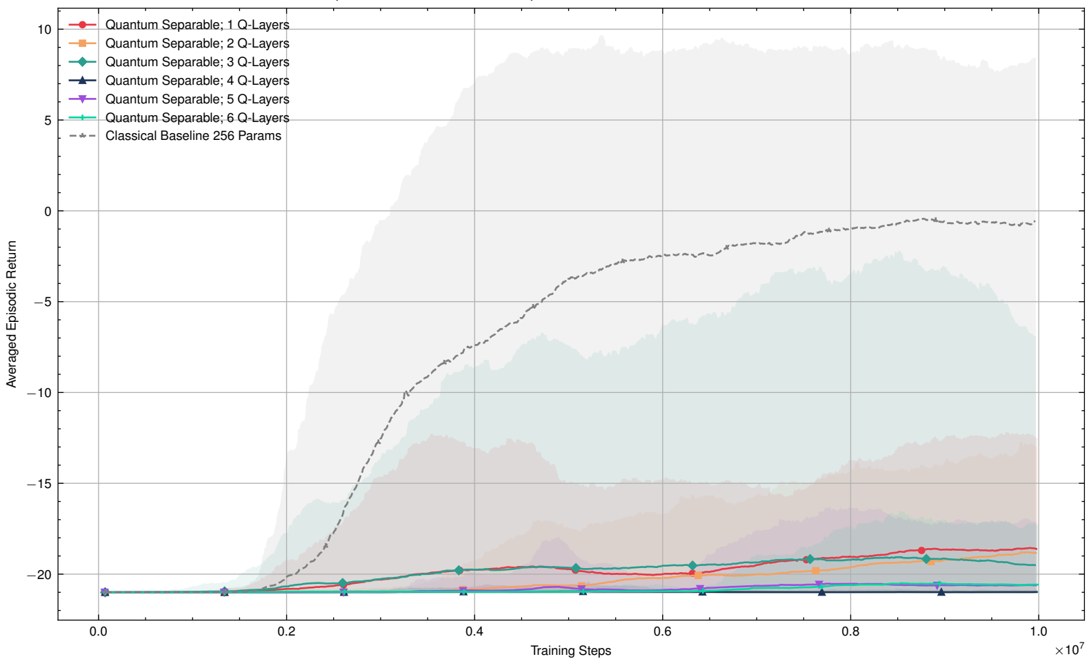
Episodic Return: Quantum Separable vs Classical Baseline 256 Params
