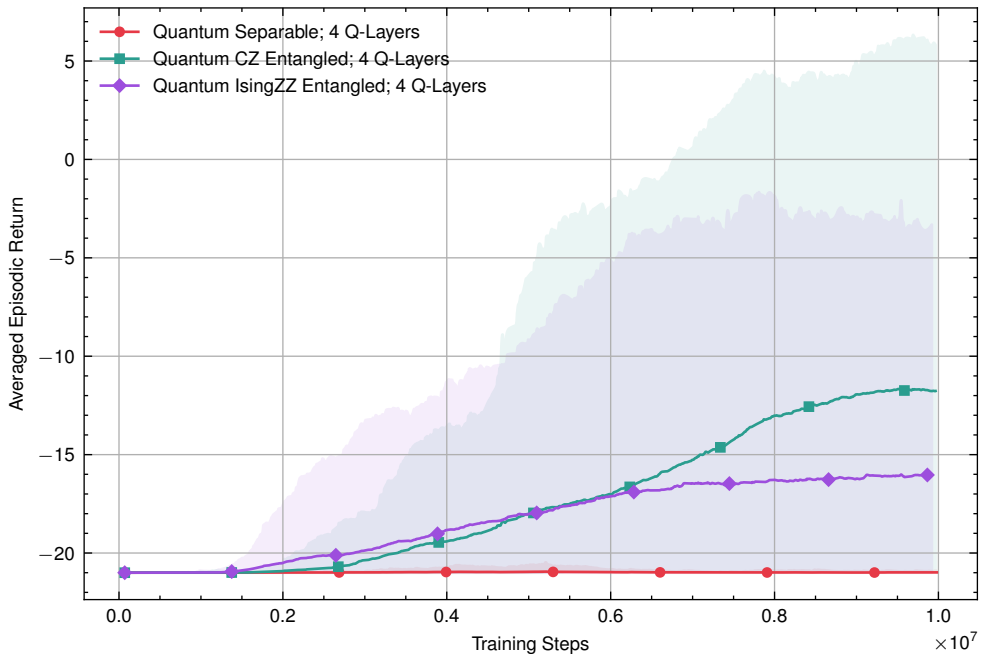
Episodic Return Comparison for 4 Q-Layers
