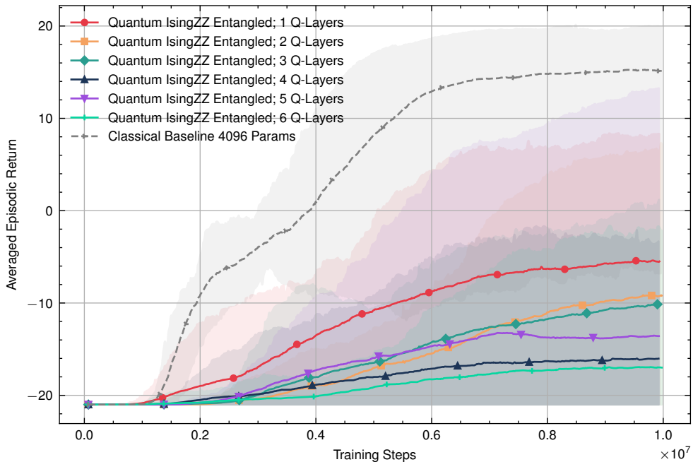
Episodic Return: Quantum IsingZZ Entangled vs Classical Baseline 4096 Params
