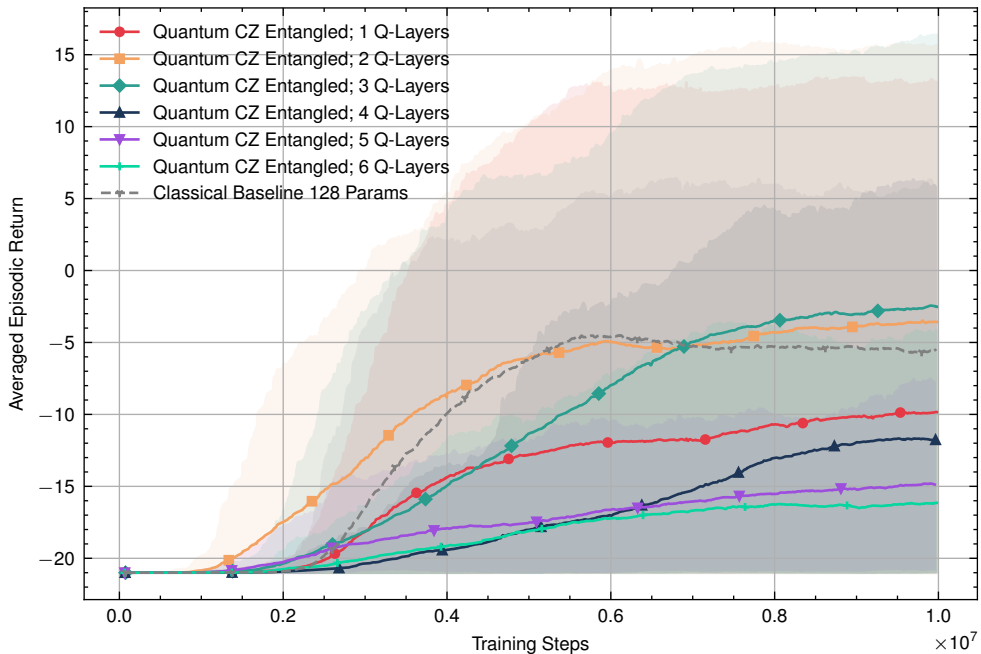
Episodic Return: Quantum CZ Entangled vs Classical Baseline 128 Params
