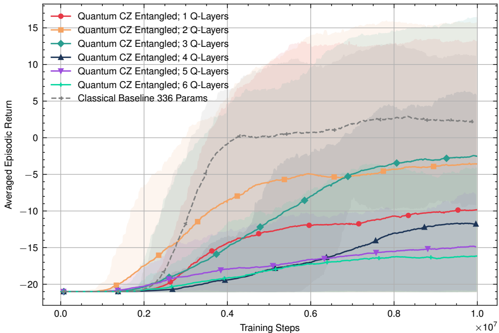
Episodic Return: Quantum CZ Entangled vs Classical Baseline 336 Params
