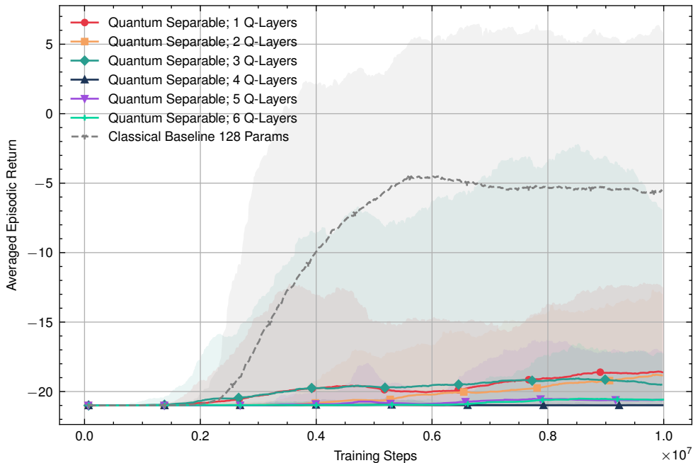
Episodic Return: Quantum Separable vs Classical Baseline 128 Params
