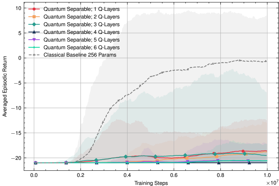
Episodic Return: Quantum Separable vs Classical Baseline 256 Params
