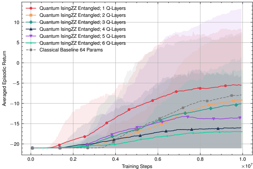
Episodic Return: Quantum IsingZZ Entangled vs Classical Baseline (64 Params)
