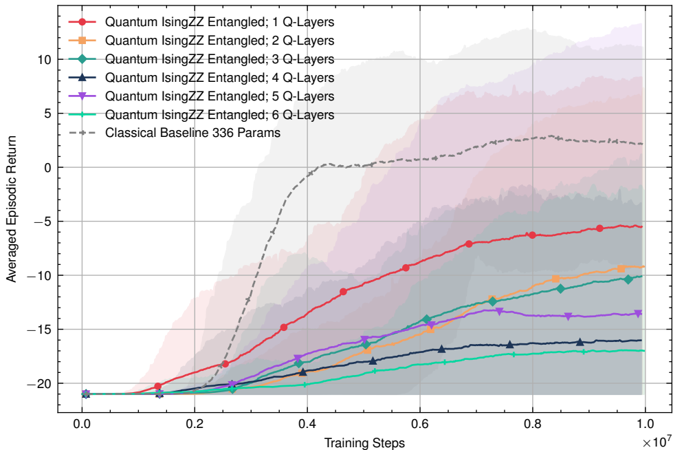
Episodic Return: Quantum IsingZZ Entangled vs Classical Baseline 336 Params
