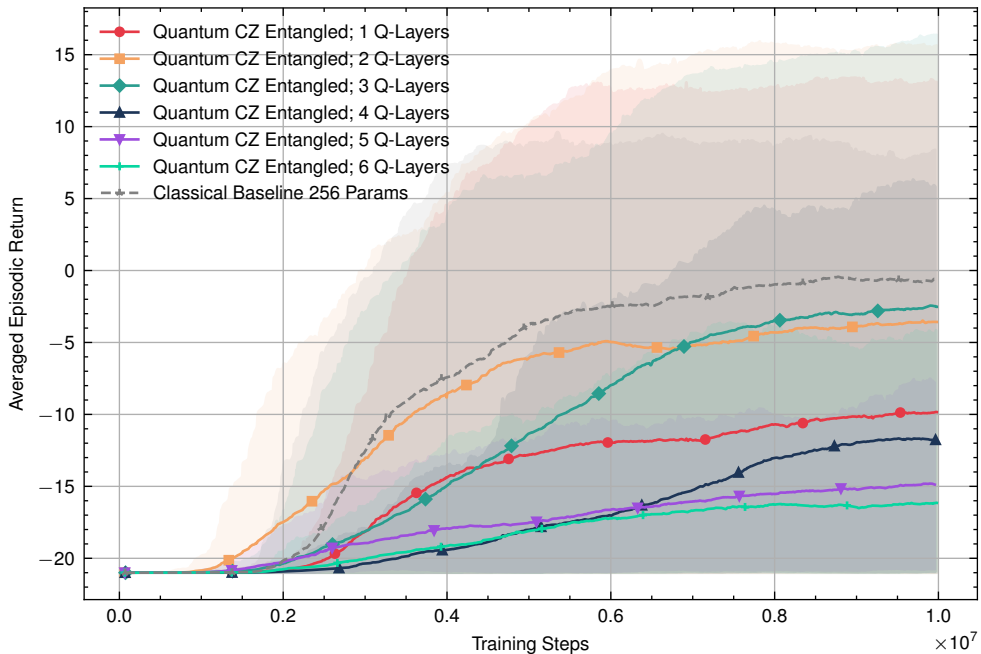
Episodic Return: Quantum CZ Entangled vs Classical Baseline 256 Params
