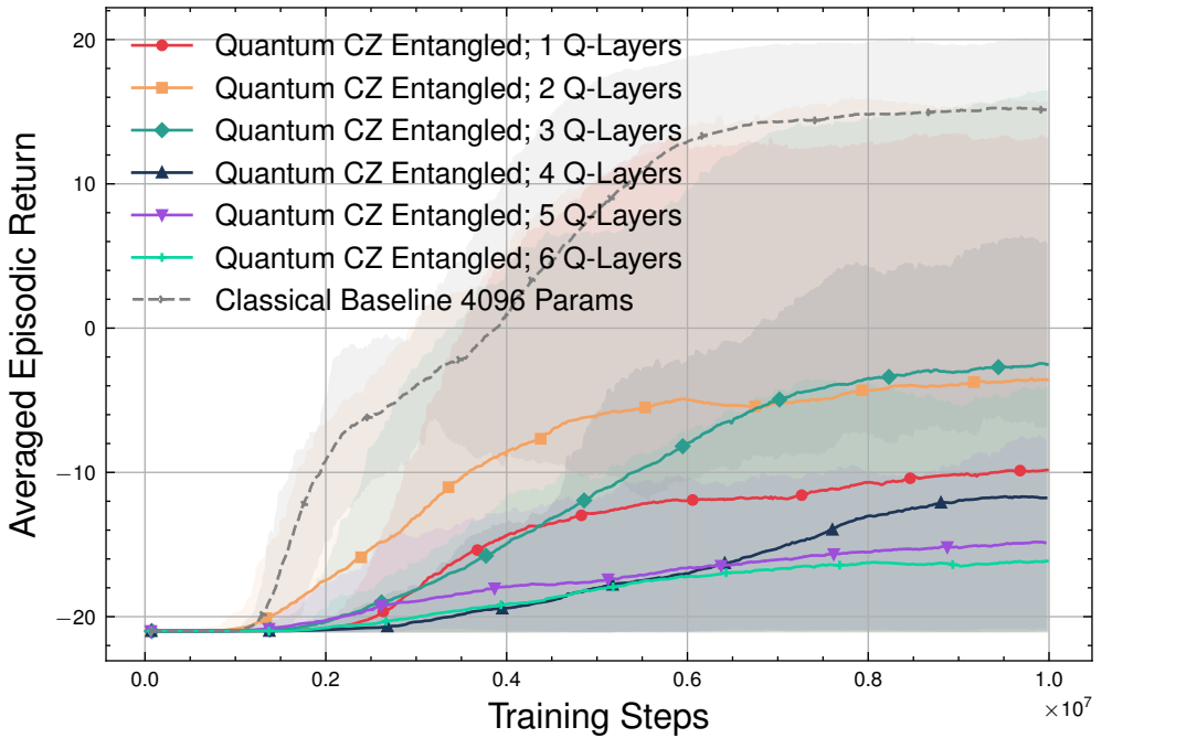
Episodic Return: Quantum CZ Entangled vs Classical Baseline 4096 Params
