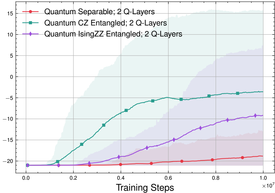
Episodic Return Comparison for 2 Q-Layers
