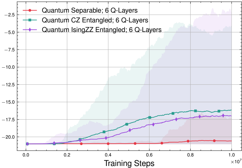
Episodic Return Comparison for 6 Q-Layers
