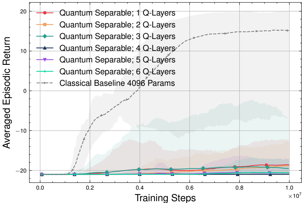
Episodic Return: Quantum Separable vs Classical Baseline 4096 Params
