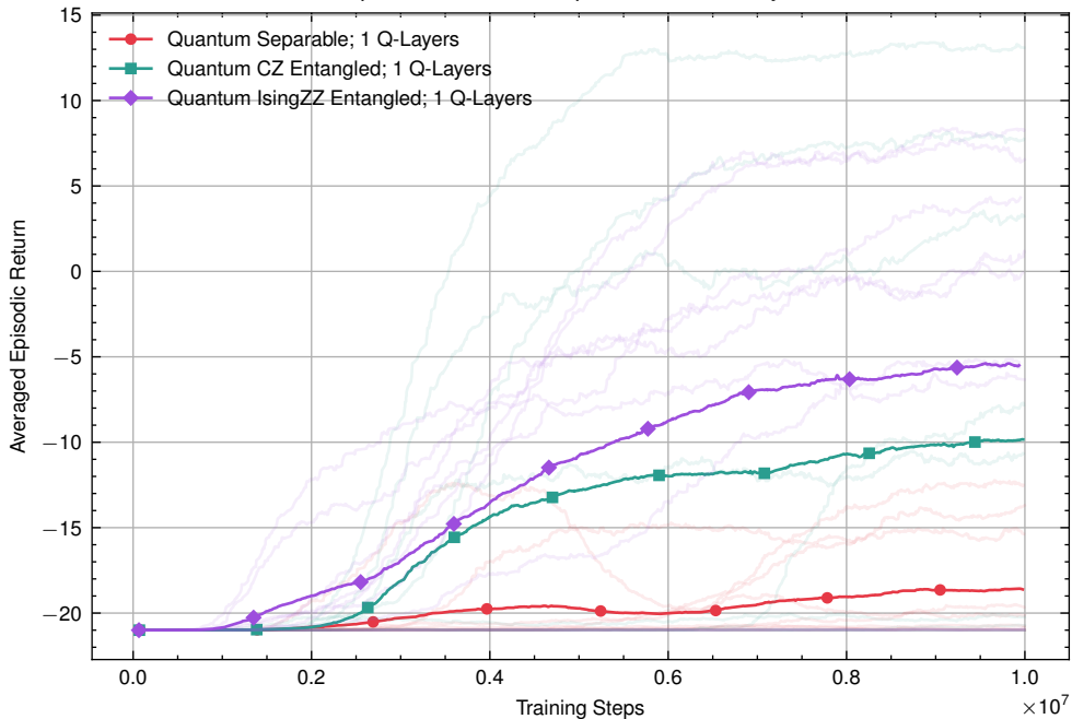
Episodic Return Comparison for 1 Q-Layers
