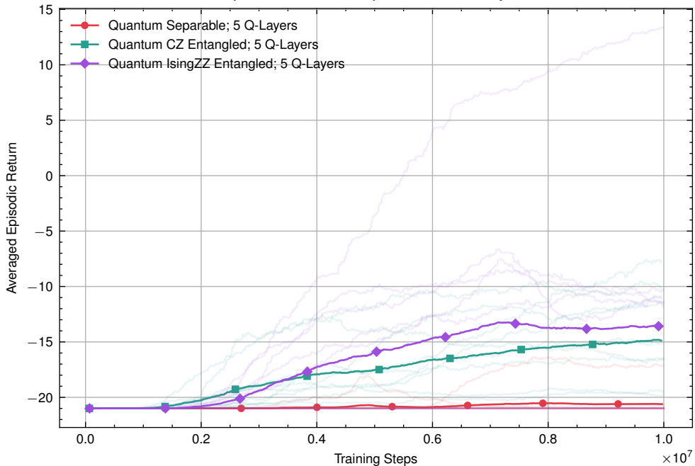
Episodic Return Comparison for 5 Q-Layers
