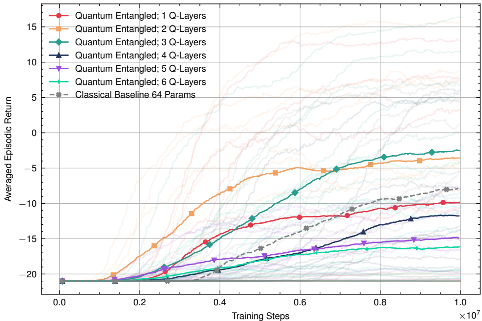
Episodic Return: Quantum CZ Entangled vs Classical Baseline (64 Params)
