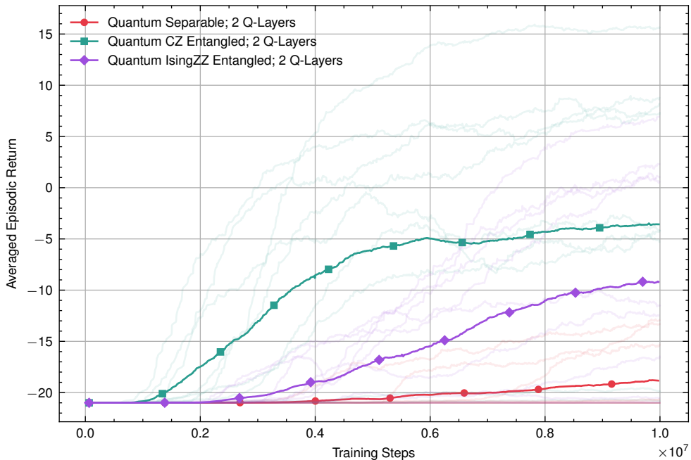
Episodic Return Comparison for 2 Q-Layers
