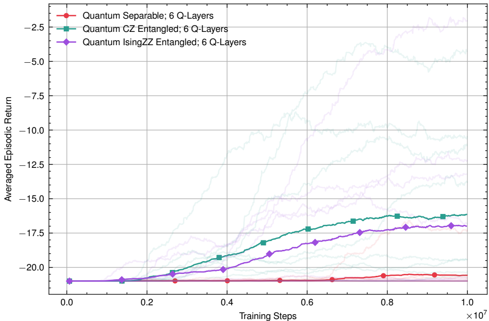
Episodic Return Comparison for 6 Q-Layers
