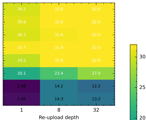
Pendigits STA4
