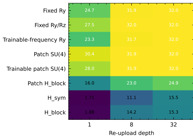
Pendigits DYN
