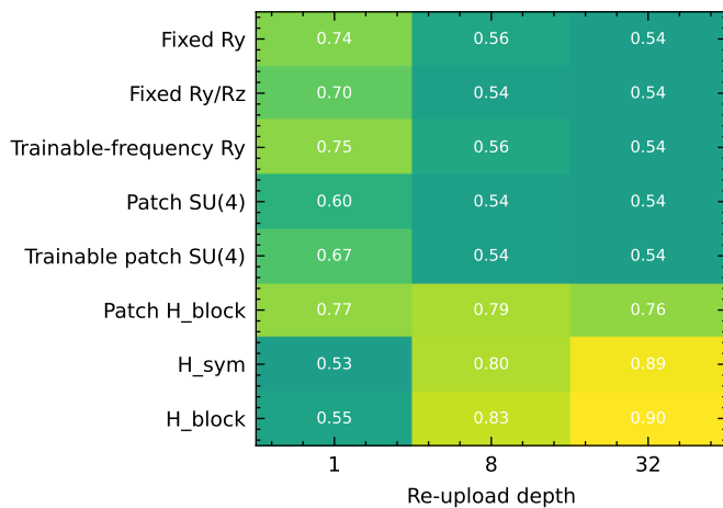
Pendigits DYN
