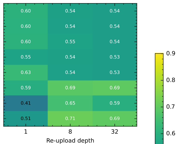
Pendigits STA4
