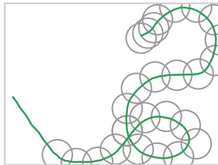
V3 TCN-WGAN
