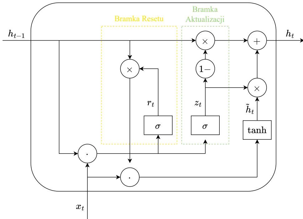
Rysunek 5. Schemat komórki GRU ( Gated Recurrent Unit ). Widoczny przepływ sygnałów przez bramkę resetu ( r_t ) oraz bramkę aktualizacji ( z_t ). Symbol \sigma oznacza funkcję aktywacji sigmoidalną, a \tanh tangens hiperboliczny. Źródło: opracowanie własne na podstawie [27].
