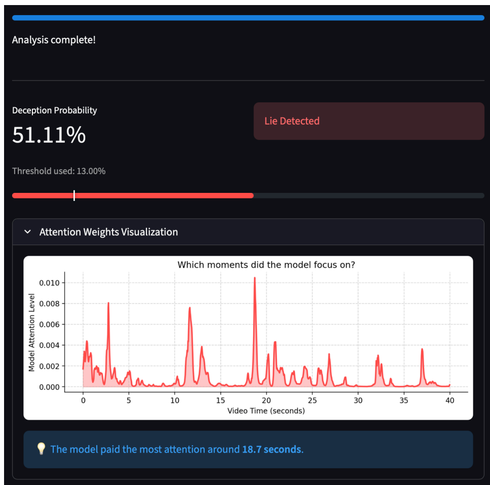
Rysunek 21. Panel wyników analizy. Widoczna ocena prawdopodobieństwa kłamstwa, wizualizacja progu decyzyjnego oraz wykres wag atencji wskazujący na podejrzone fragmenty nagrania.
