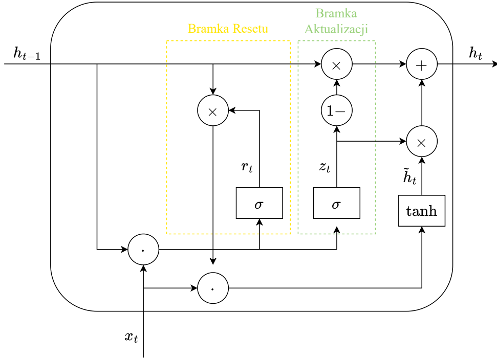
Rysunek 5. Schemat komórki GRU ( Gated Recurrent Unit ). Widoczny przepływ sygnałów przez bramkę resetu ( r_t ) oraz bramkę aktualizacji ( z_t ). Symbol \sigma oznacza funkcję aktywacji sigmoidalną, a \tanh tangens hiperboliczny. Źródło: opracowanie własne na podstawie [32].
