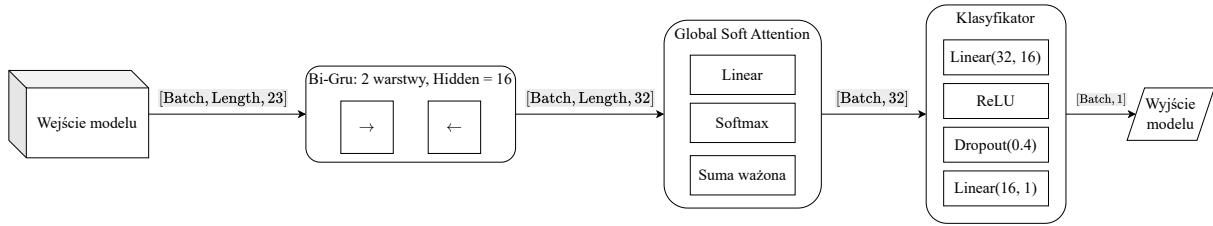
Rysunek 8. Schemat architektury modelu BiGRU z mechanizmem uwagi. Wymiary tensorów podano w nawiasach kwadratowych nad strzałkami przepływu danych.
