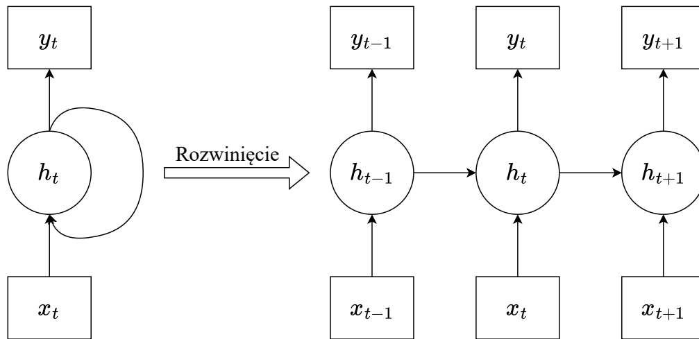
Rysunek 4. Schemat sieci rekurencyjnej (RNN). Po lewej: reprezentacja zwinięta z pętlą sprzężenia zwrotnego. Po prawej: reprezentacja rozwinięta w czasie, ukazująca przepływ informacji (stanu ukrytego) przez kolejne kroki sekwencji. Źródło: opracowanie własne na podstawie [29].
