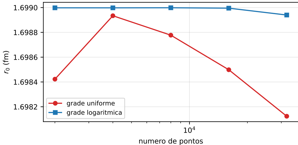
Lennard-Jones: convergencia de r_0
