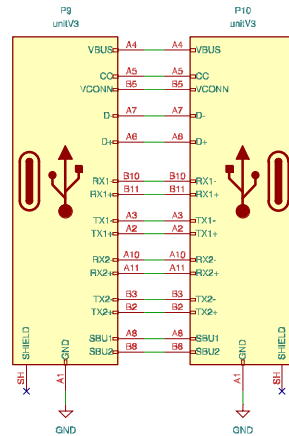
Connector_unitV3
