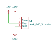
Voltmeter
