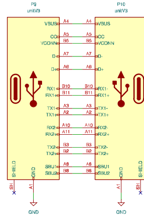
Connector_unitV3
