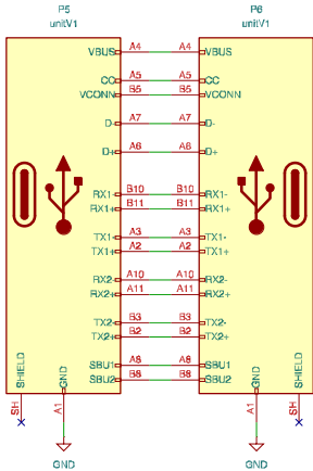
Connector_unitV1
