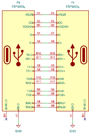
Connector_ESP32C3 2
