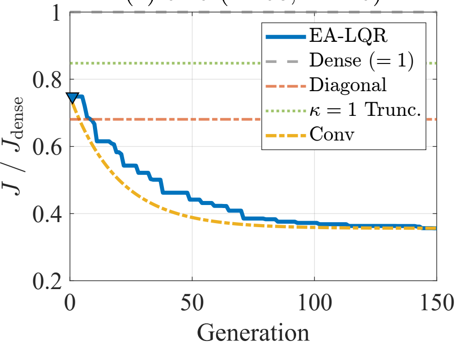
(d) 5 \times 5 EA controller
