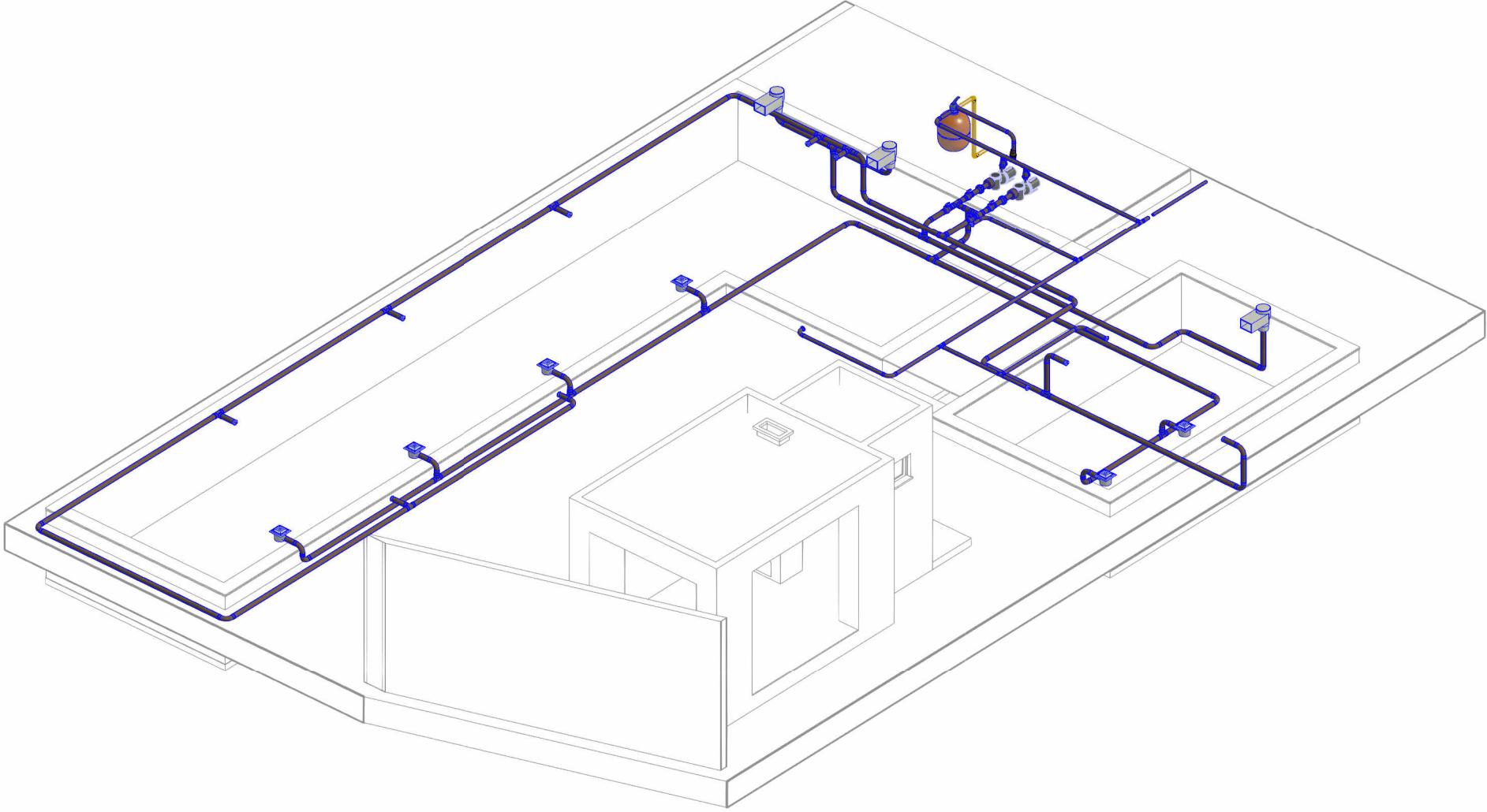
Isométrico Piscina
