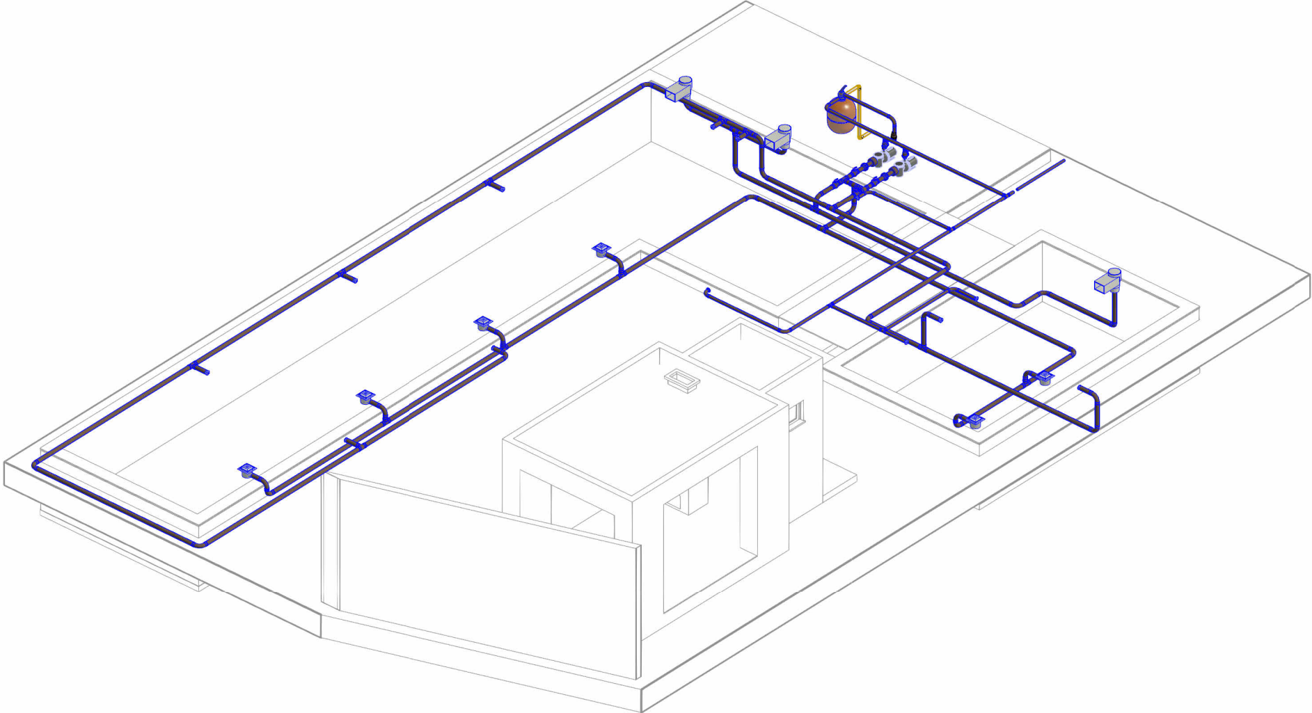
Isométrico Piscina
