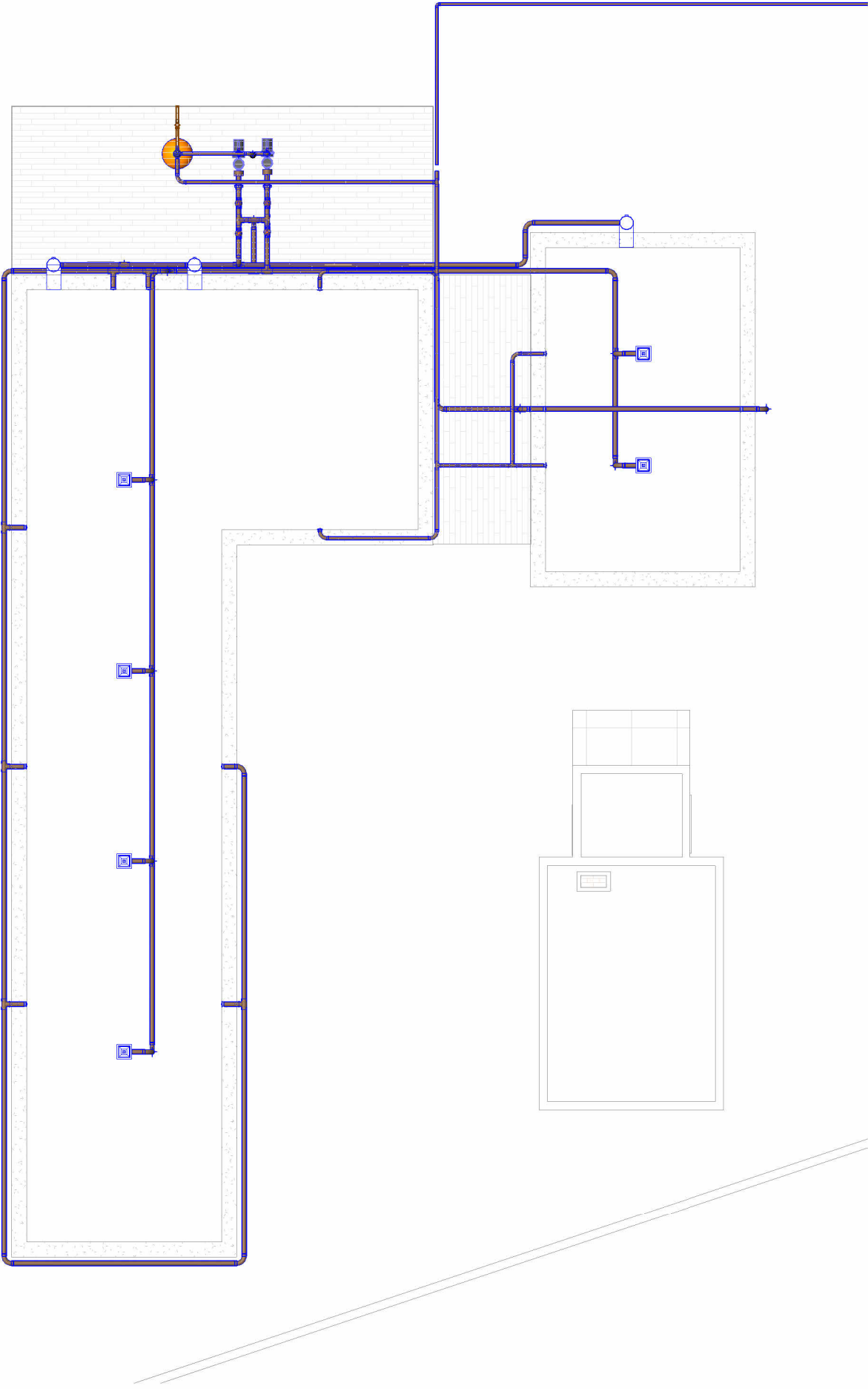
Planta Baixa Piscina 1 : 100
