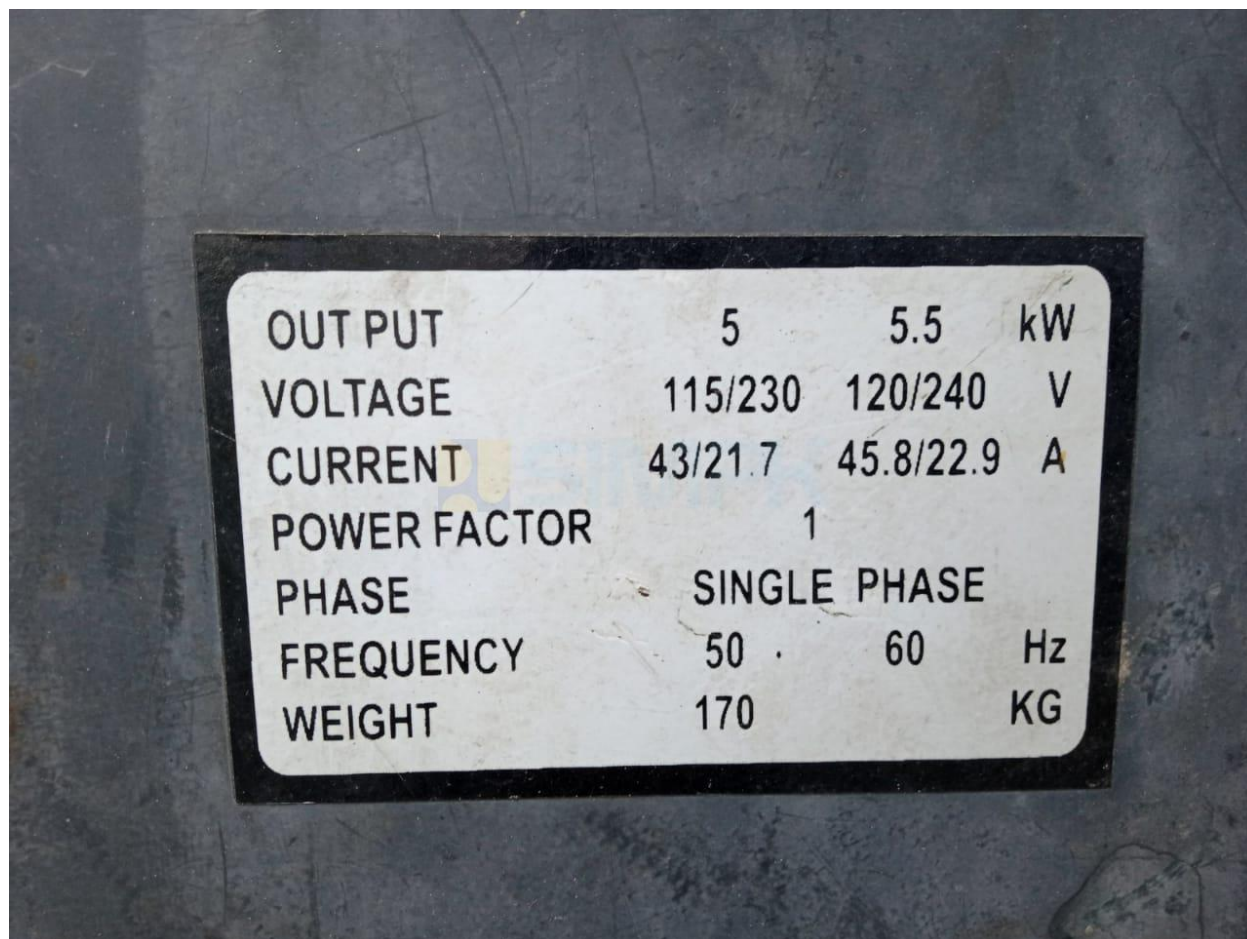
Contoh Foto Plat Generator Set
