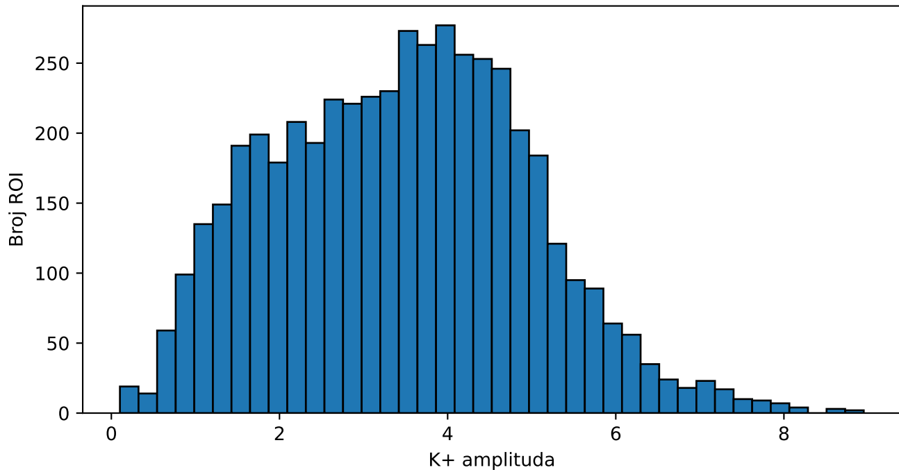
Raspodela K+ amplitude (svi eksperimenti)
