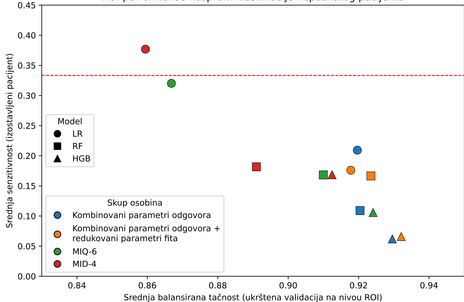
ROI performanse naspram klasifikacije nepoznatog pacijenta
