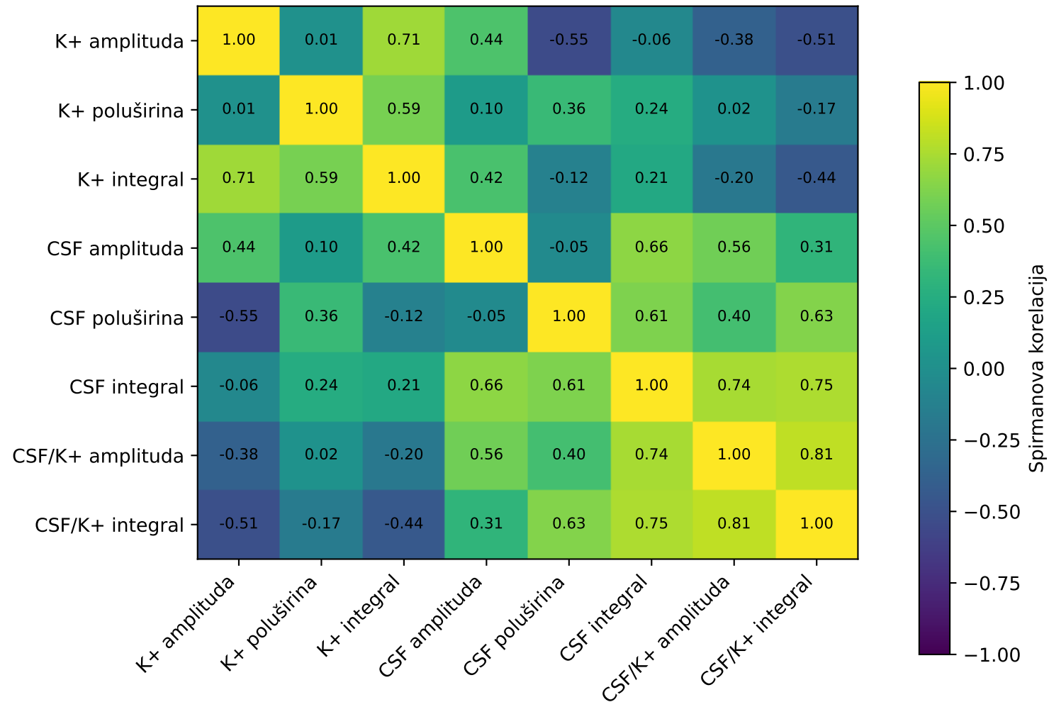
ROI sa detektovanim CSF odgovorom
