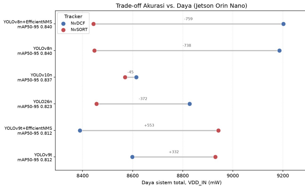
Diagram pasangan ( dumbbell ) trade-off akurasi mAP50-95 versus daya sistem total: satu baris per model diurutkan menurut akurasi, titik NvDCF dan NvSORT dihubungkan garis yang panjangnya menunjukkan selisih daya akibat pergantian tracker
