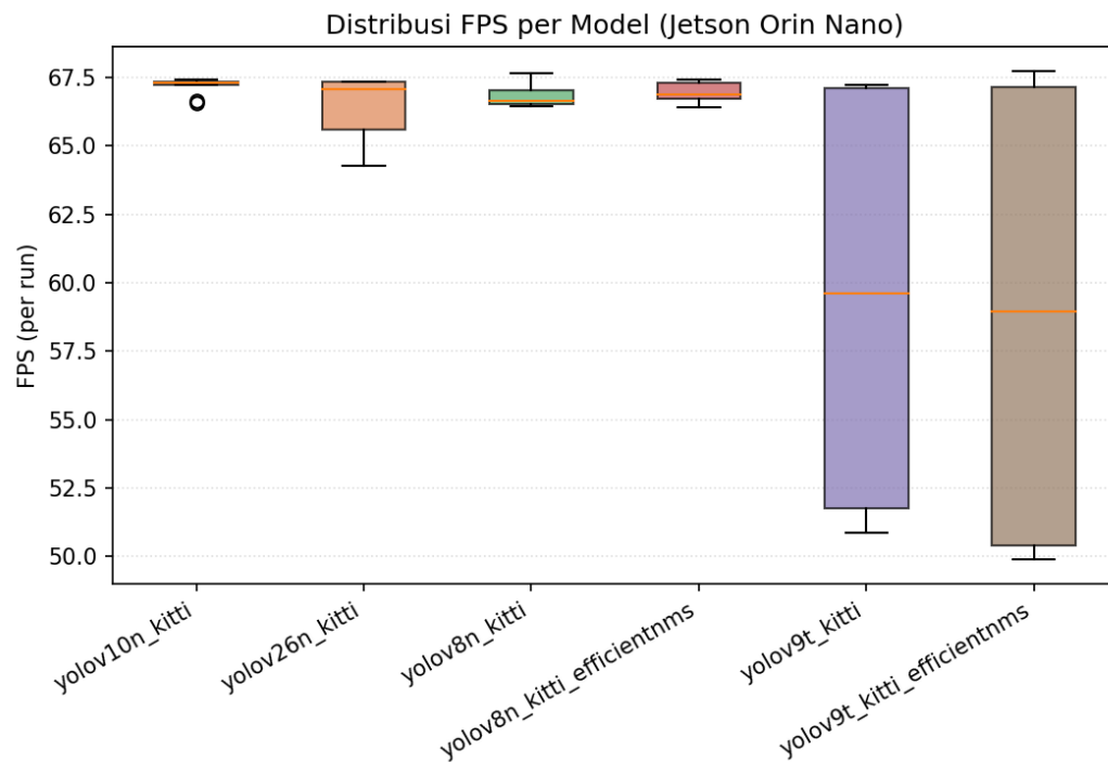
Distribusi FPS per model, digambarkan sebagai kotak-garis (boxplot) yang merangkum rentang, median, dan sebaran seluruh run per model
