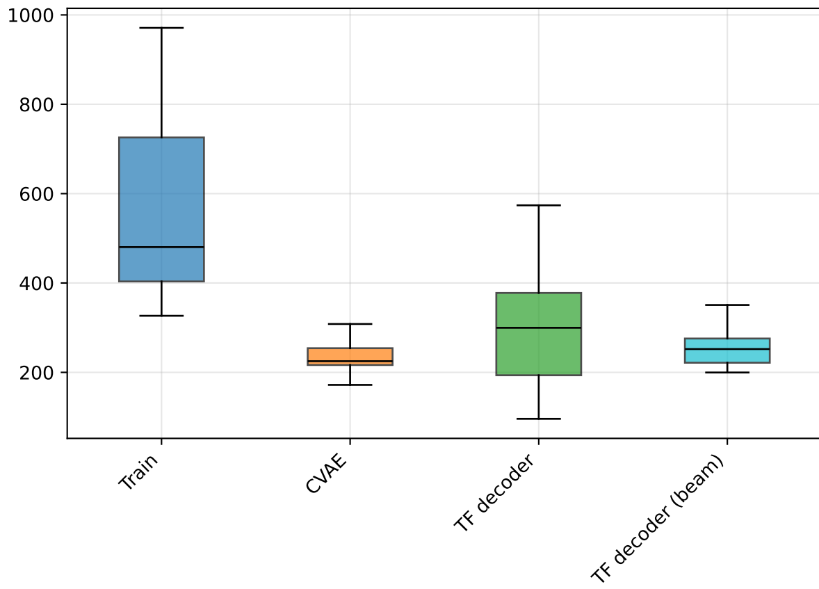
CTD - SEPSIS
