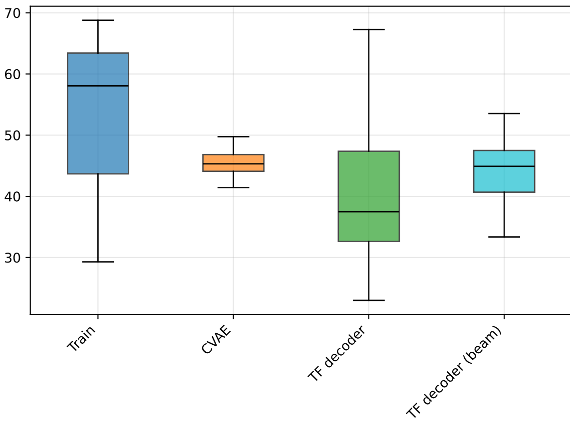
CTD - SEPSIS
