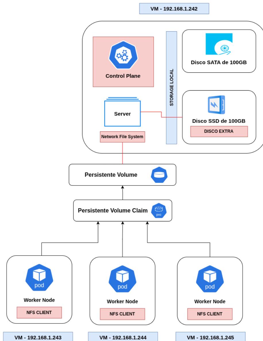
Figura 9 – Cenário 01: Cluster com NFS
